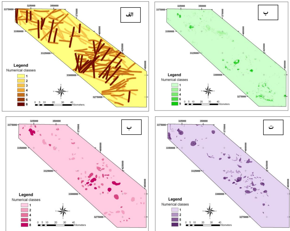
شکل ۳-۳- نقشه‌های نشانگر عددی برای لایه‌های الف) ساختاری، ب) ژئوشیمیایی، پ) دگرسانی و ت) ژئوفیزیکی
